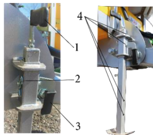
Rys.23. 1. Rączka do ustawienia wys. stopki. 2. Zawleczka zabezpieczająca. 3. Sworzeń z uchwytem. 4. Otwory do ustawienia wysokości stopki.
