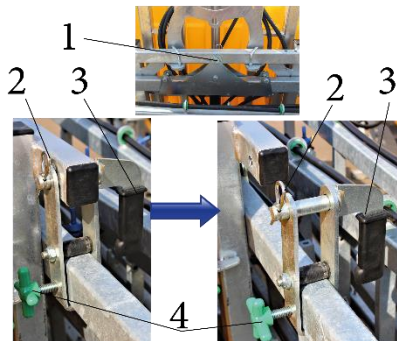
Rys.28. Budowa grawitacyjnej stabilizacji belki polowej. 1. Sworzeń centralny. 2. Zawleczka zabezpieczająca. 3. Rączka blokady stabilizacji. 4. Śruba unieruchamiająca blokadę.
