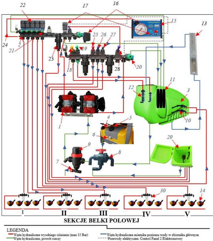
Rys.54. 1. Pompa Tandem Tolver® PU-3/140. 2. Rozdzielacz sterujący. 3. Zbiornik główny. 4. Zbiornik na wodę do mycia układu. 5. Zbiornik na wodę do mycia rąk. 6. Kranik ON/OFF zbiornika do mycia rąk. 7. Zawór spustowy. 8. Zawór trójdrożny do sterowania zasysaniem cieczy z poszczególnych zbiorników. 9. Filtr ssawny. 10. Mieszadła hydrauliczne antypieniące. 11. Węże hydrauliczne zapobiegające pienieniu się cieczy roboczej krążącej w obiegu. 12. Rozwadniacz nawozów stałych. 13. Miernik zawartości wody w zbiorniku głównym. 14. Głowica obrotowa z rozpylaczami. 15. Control Panel 2®. 16. Elektrozwór włącz/wyłącz sterowany poprzez Control Panel 2®. 17. Elektrozwór do sterowania ciśnieniem rozpylaczy poprzez Control Panel 2®. 18. Dźwignia rozwadniacza sitowego. 19. Dźwignia do mycia zbiornika głównego. 20. Regulator ciśnienia doprowadzanego do rozdzielacza sterującego. 21. Zawór kompensacyjny ciśnienia sekcji. 22. Elektrozawór sekcji. 23. Filtr ciśnieniowy. 24. Przewód manometru podłączany do Control Panel 2®. 25. Dźwignia mieszadła. 26. Dźwignia do napełniania rozwadniacza bocznego. 27. Dźwignia rozwadniacza bocznego od mycia butelek. 28. Dźwignia zasilająca rozwadniacz boczny. 29. Rozwadniacz boczny. 30. Filtr liniowy
