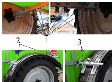
Rys.35. 1. Śruby mocujące oś. 2. Uchwyty mocowania błotników. 3. Śruby mocowań błotników
