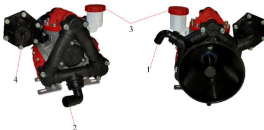
Rys.44. Pompa Tolveri PU-3/140. 1 Króciec tłoczny. 2. Króciec ssawny. 3. Wlew oleju wraz z kontrolą poziomą. 4. Wentyl powietrznika. Prawidłowe ciśnienie 1/3 ciśnienia roboczego pompy- nie więcej niż 105 Bar.
