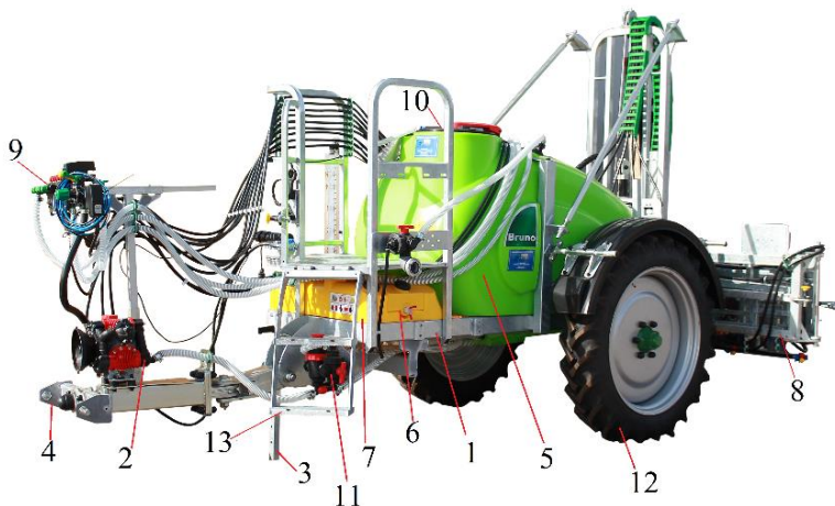
Rys.3. 1. Rama główna. 2. Pompa. 3. Podpora. 4. Belka zaczepowa. 5. Zbiornik główny. 6. Zbiornik na wodę do mycia rąk. 7. Zbiornik na wodę do mycia układu. 8. Belka polowa.
