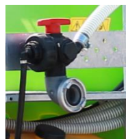
Rys. 16. Hydrant
