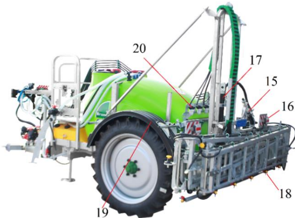
Rys.4. 15. Stabilizacja belki. 16. Światła z tablicami ostrzegawczymi. 17. Siłownik do regulacji wysokości pracy belki polowej. 18. Głowica rozpylacza. 19. Błotnik. 20. Filtr liniowy
