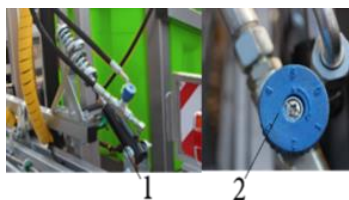
Rys.29. Stabilizacja hydrauliczna belki polowej rozkładanej ręcznie. Opis 1. Siłownik hydrauliczny. 2. Pokrętło regulacji.
