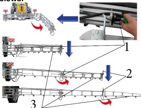
Rys.27. Otwieranie ręcznej piętnastometrowej belki polowej w opryskiwaczu „Bruno”. 1. Zabezpieczenie niezatraskowe. 2. Zabezpieczenie sprężynowe. 3. Miejsca do uchwycenia podczas rozkładania belki.
