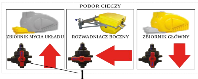
Rys. 31. Obsługa zaworu czterodrożnego. 1. Pokrętko.
