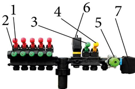
Rys. 33. Rozdzielacz sterujący w podstawowej wersji. 1. Dźwignia sekcji belki polowej. 2. Pokrętło kalibracji ciśnienia. 3. Dźwignia rozwadniacza. 4. Dźwignia do mycia zbiornika głównego. 5. Główny zawór regulacji ciśnienia. 6. Elektrozwór regulacji ciśnienia. 7. Elektrozwór włącz/wyłącz.
