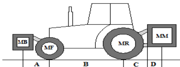
Rys.3. Określenie stateczności statycznej
