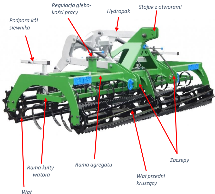
Zdj.2. Budowa agregatu uprawowo- siewnego
