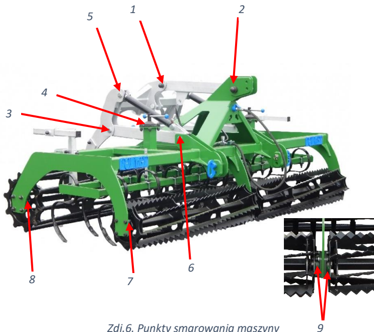
Zdj.6. Punkty smarowania maszyny
