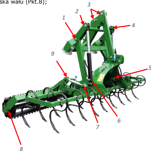
Zdj.4. Punkty smarowania maszyny
