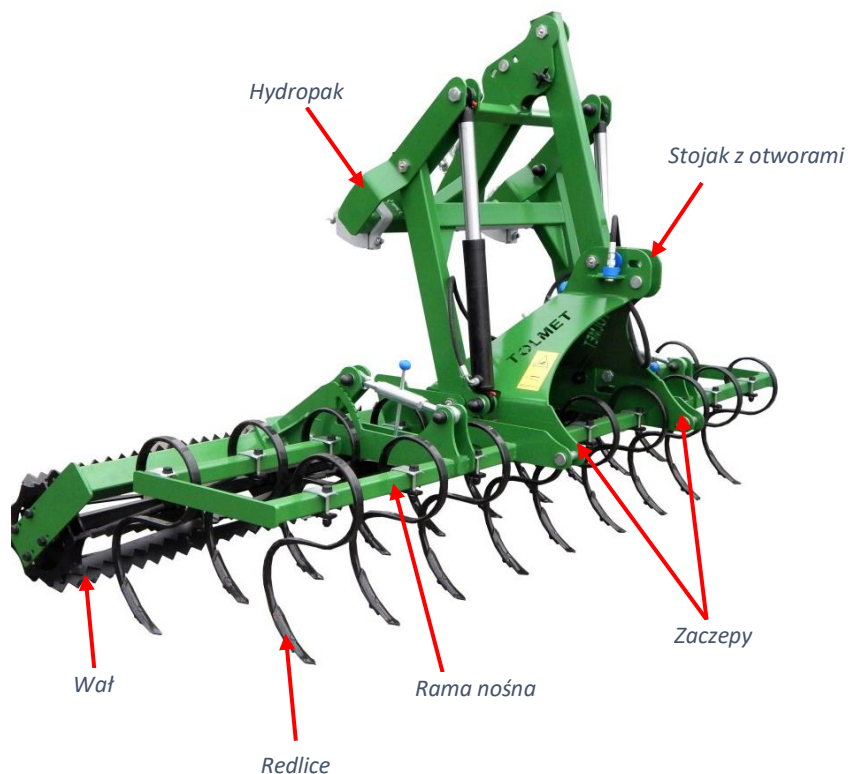
Zdj.2. Budowa agregatu uprawowo-siewnego
