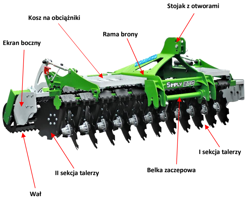
Zdj.2. Budowa brony kompaktowej Simply
