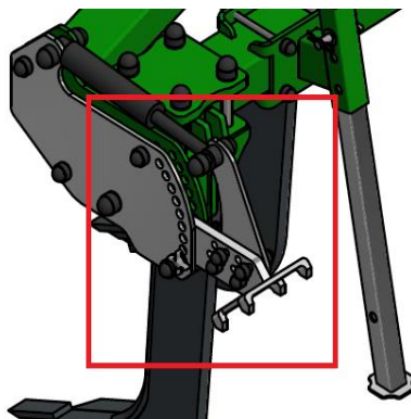
Zdj.10. Regulacja ucha siłownika
