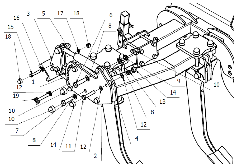
Rys.11.Ramiona wału z hydrauliką.
