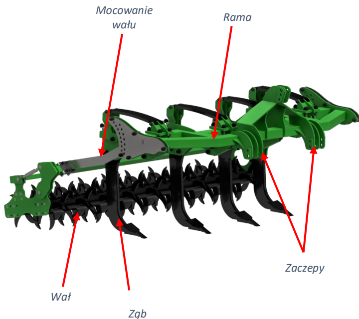
Zdj.2. Budowa głębosza
