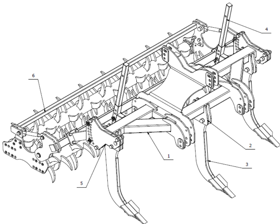
Rys.1.Głębosz- budowa.
